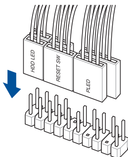
安装系统控制面板接口
